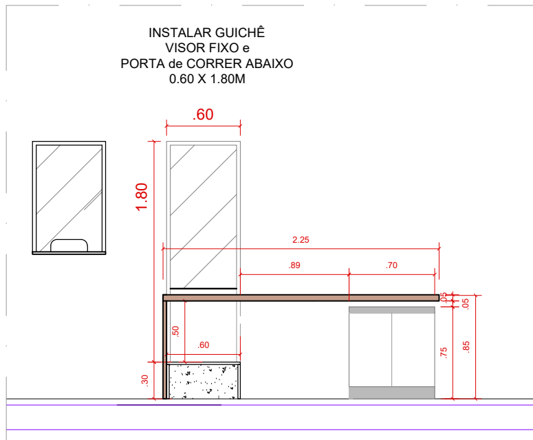
VISTA
