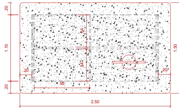
PLANTA BAIXA - TAMPO NANOGLASS
