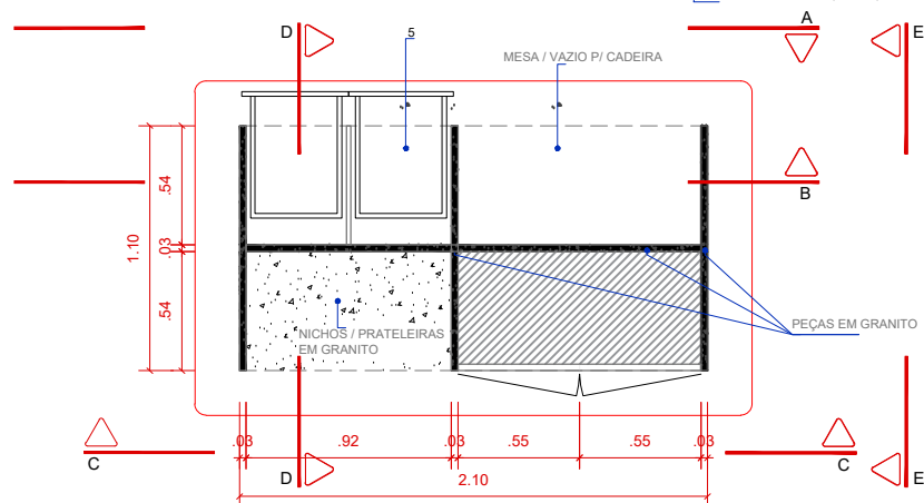
PLANTA BAIXA
