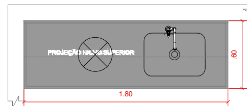
BANCADA DE INOX - VISTA SUPERIOR
