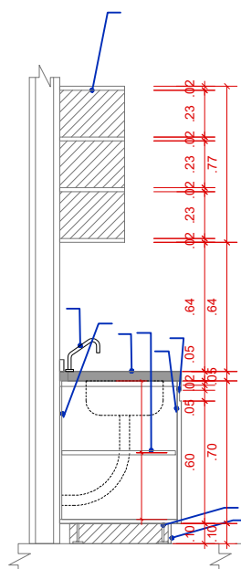
CORTE BB
