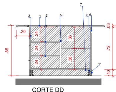
CORTE DD
