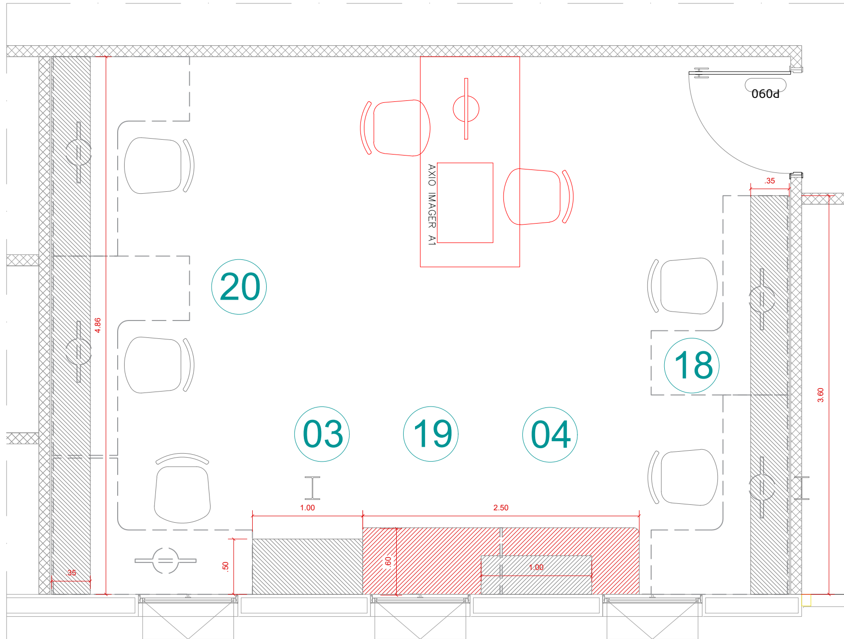
LAUDO-PATOLOGIA E MICROSCOPIA - PLANTA BAIXA
