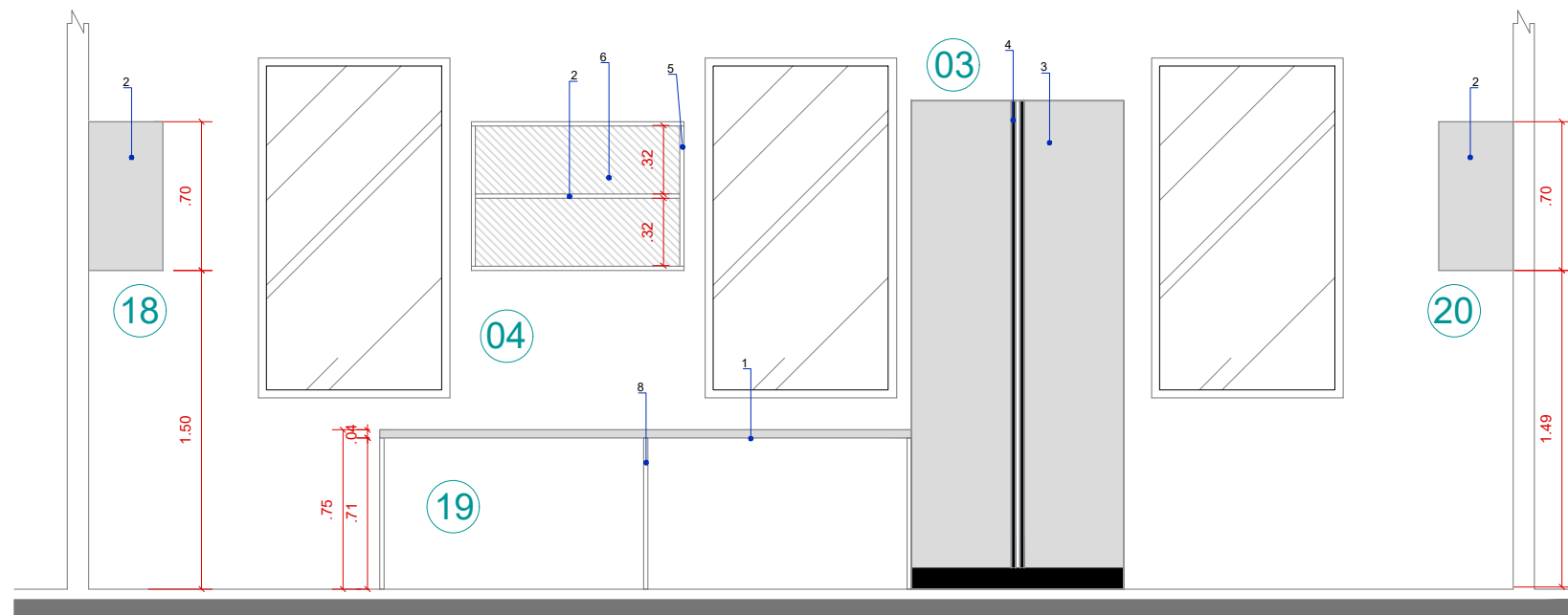
VISTA 01- FRONTAL
