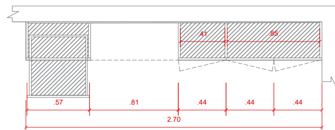
PLANTA BAIXA ARMÁRIO AÉREO
