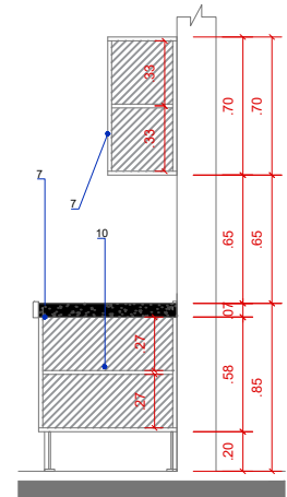
CORTE BB
