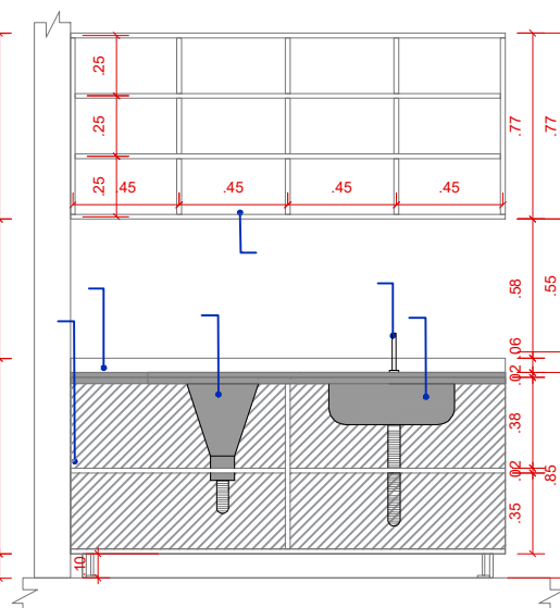
CORTE AA
