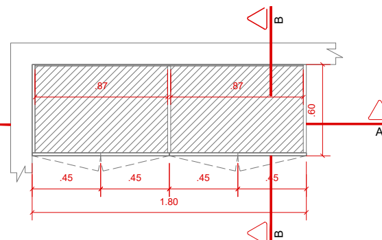
PLANTA BAIXA - ARMÁRIO OBS. CONSIDERAR INSTALAÇÕES DE EXPURGO E DA CUBA PARA EXECUTAR A MARCENARIA, CONFERIR MEDIDAS DAS MESMAS NO LOCAL
