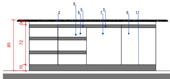
VISTA FRONTAL AA BANCADA TIPO ILHA
